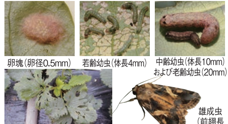
卵塊(卵径0.5mm) 若齢幼虫(体長4mm) 中齢幼虫(体長10mm) および老齢幼虫(20mm) 雄成虫(前翅長18mm)
